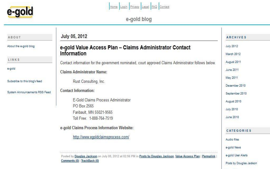
Gambar 3.1 : Tampilan E-Gold
