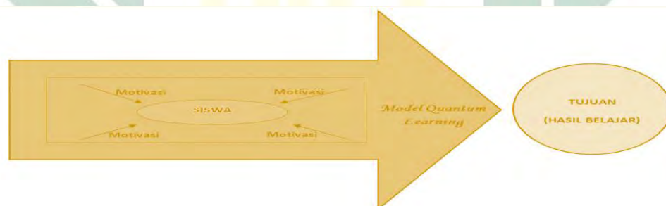
Gambar 2.3 Pembelajaran kuantum
