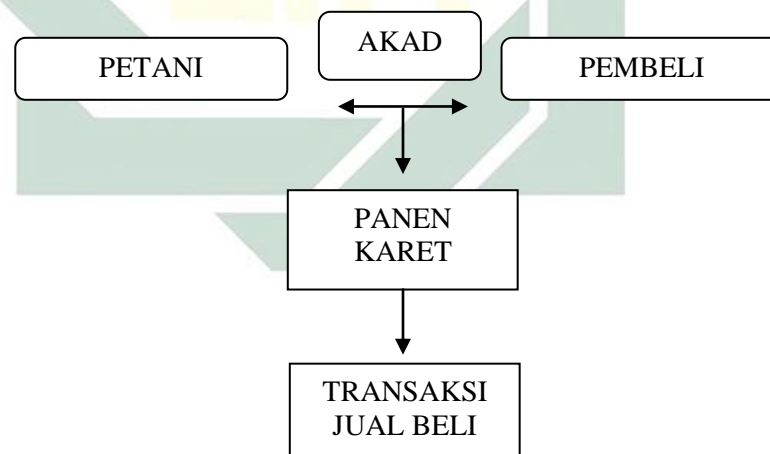
Gambar 3.2 Diagram Alur Transaksi Jual Beli Karet di Lingkungan Ujung Lombang
